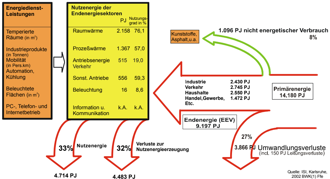
Abbildung 1: Die Energieverluste im Energienutzungssystem in Deutschland 2000
